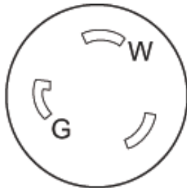
Figure 2. Prise à verrouillage par rotation L5-30R : 120 volts, 30 A
